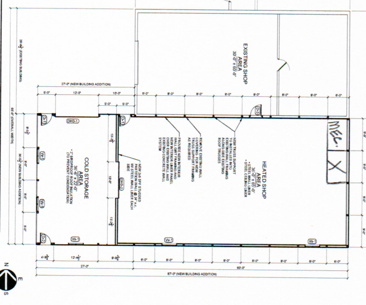
FLOOR PLAN SCALE: 1/8" = 1'-0"
