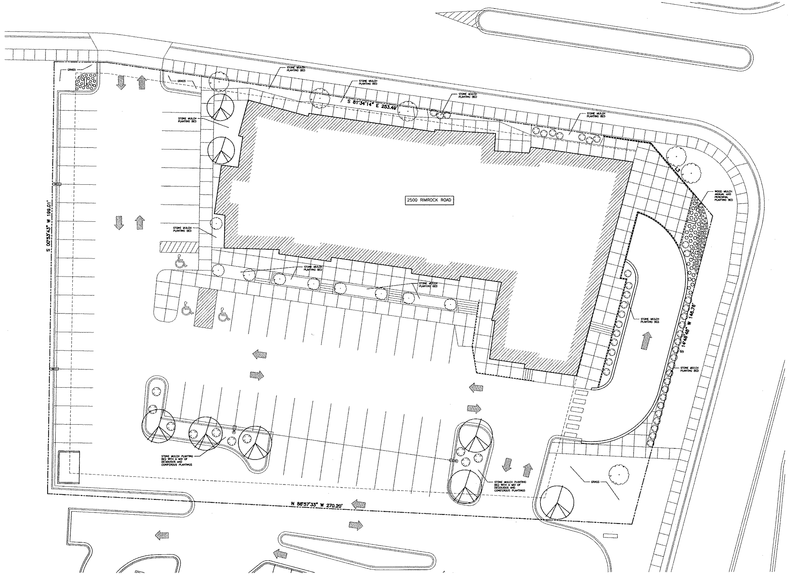
1 LANDSCAPE PLAN SCALE: N.T.S.
