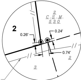
DETAIL SCALE: 1" = 5'
